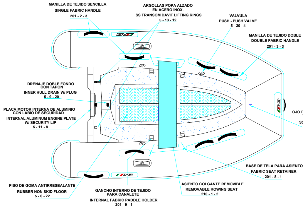
PLANT VIEW VISTA EN PLANTA
